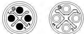
4PIN S-Coding
