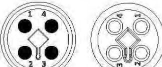
4PIN T-Coding
