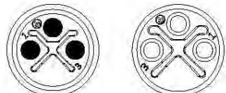
3PIN S-Coding
