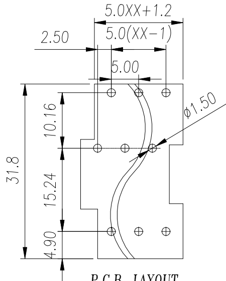
P.C.B. LAYOUT
