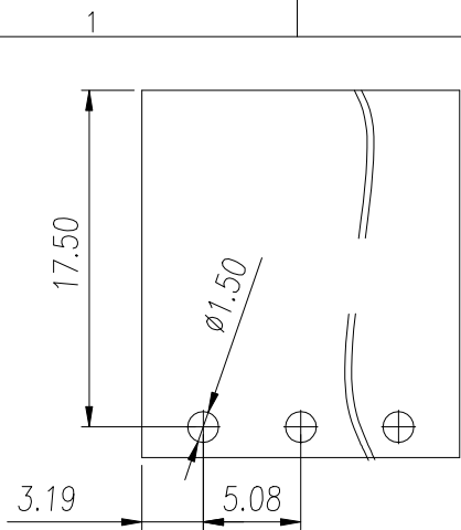
P.C.B. LAYOUT
