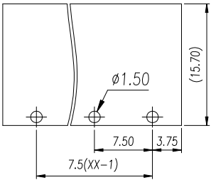
P.C.B. LAYOUT
