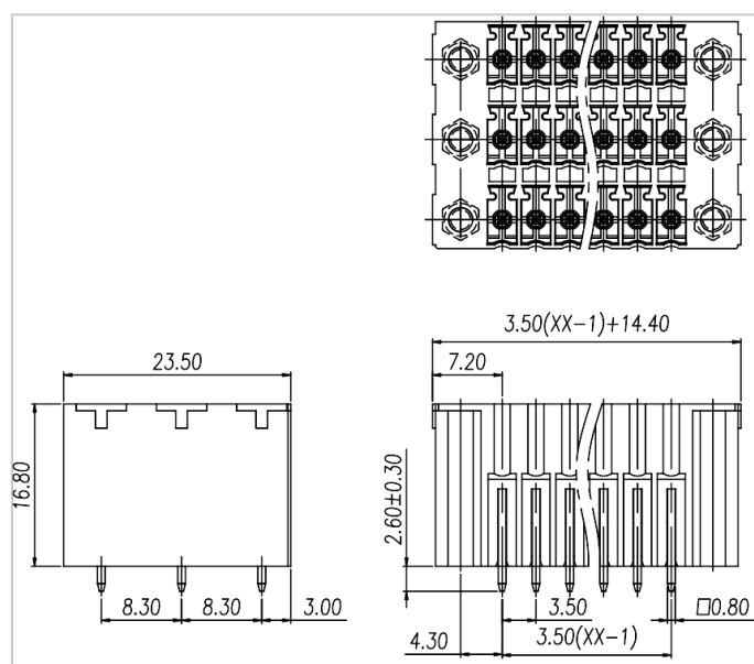
尺寸图
