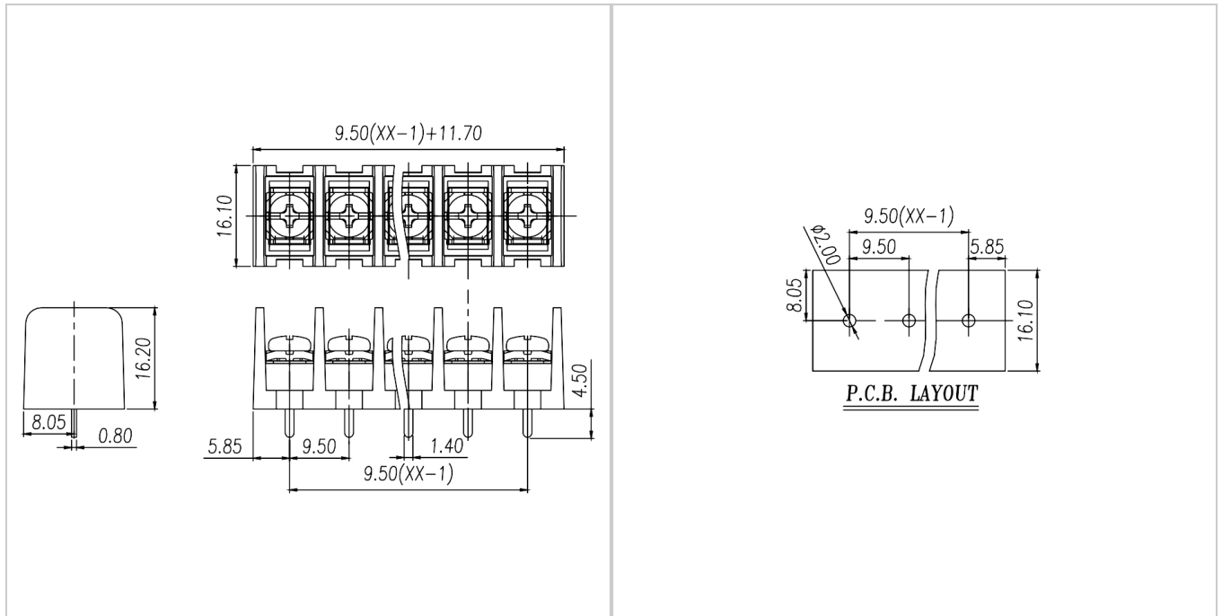
尺寸图
