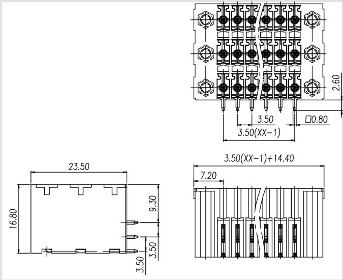
尺寸图
