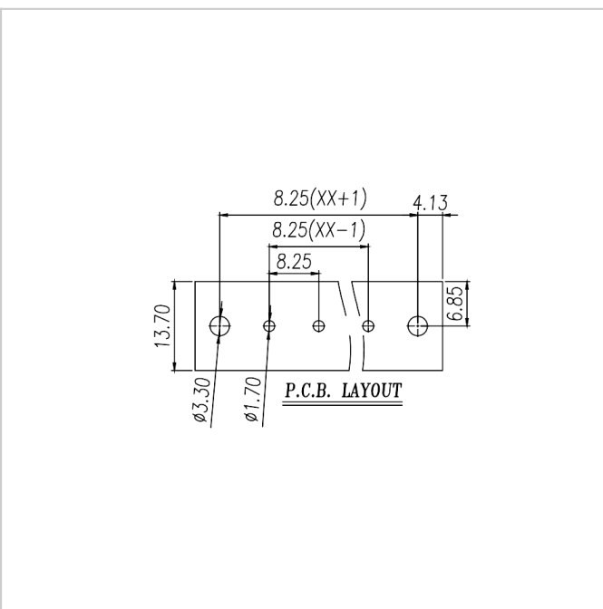
PCB开孔图
