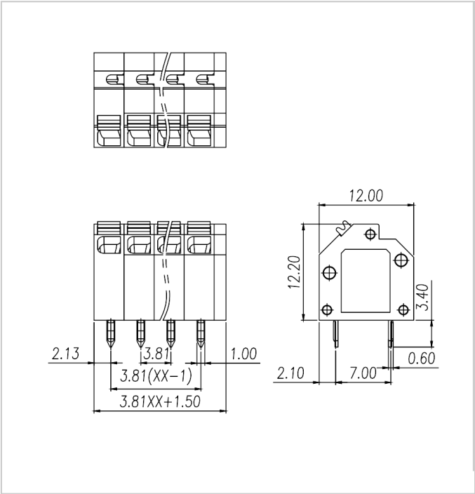
尺寸图
