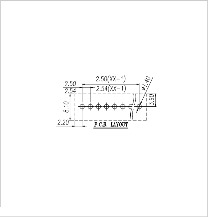
PCB开孔图
