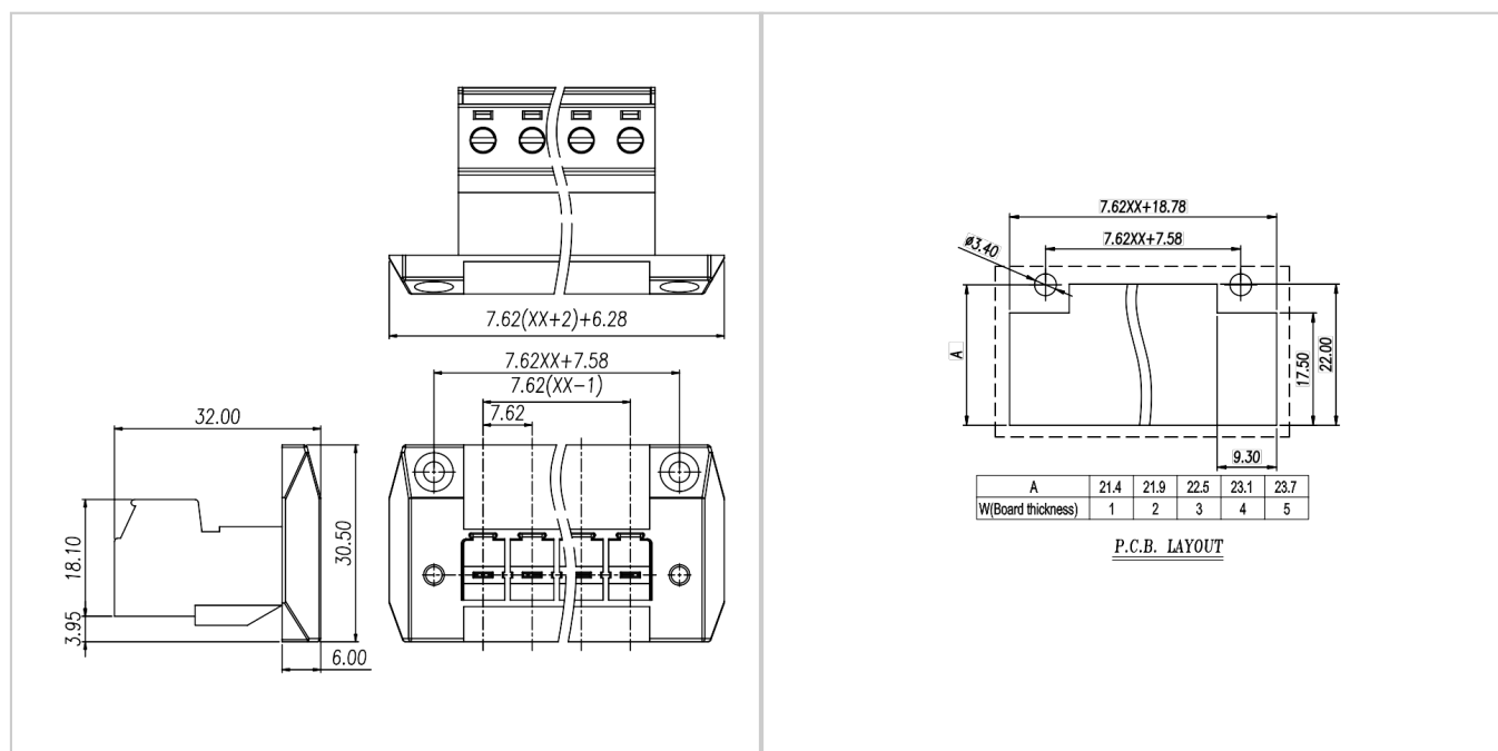
PCB开孔图
