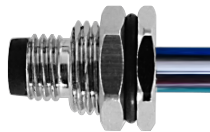
M8 公头面板式，焊接型，后锁安装，焊 M8 公头面板式，焊接型，前锁安装，焊 电子线 电子线
