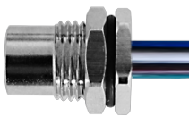
M8 母头面板式，焊接型，前锁安装，焊电子线
