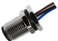
M12 公头面板式，焊接式，后锁安装
